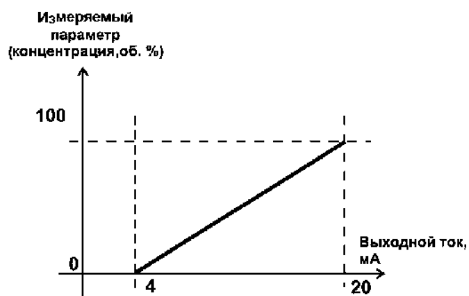
Рисунок 6.29 Пример настройки линейного выхода
