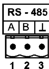
Рисунок 3.8 Вид разъема RS-485
