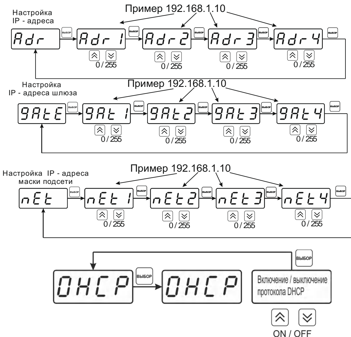
Рисунок 6.11 Сетевые настройки
