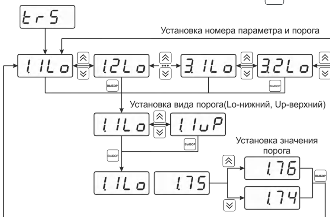
Рисунок 6.17 Задание порогов
