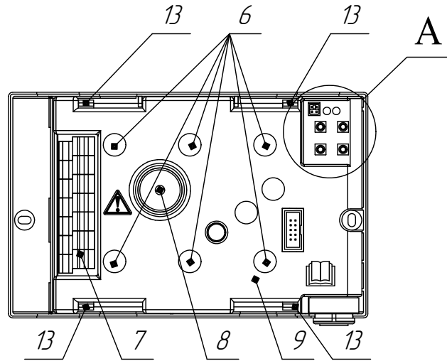
Вид спереди со снятой передней панелью
