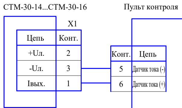
Схема подключения сигнализаторов СТМ-30-14...СТМ-30-16 к пультам контроля
