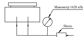
Схема гидравлических испытаний клеевых швов датчика ИБЯЛ.413226.065
