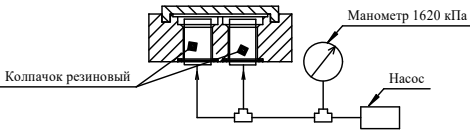
Схема гидравлических испытаний клеевых швов датчика ИБЯЛ.413226.023
