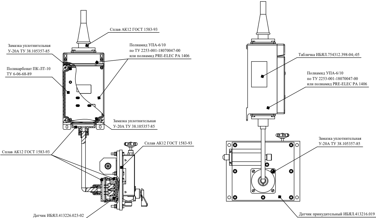
Блок датчика принудительный ИБЯЛ.413216.021;-01
