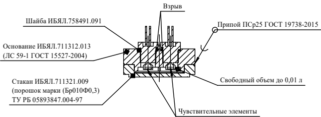
Датчик ИБЯЛ.413226.023-01
