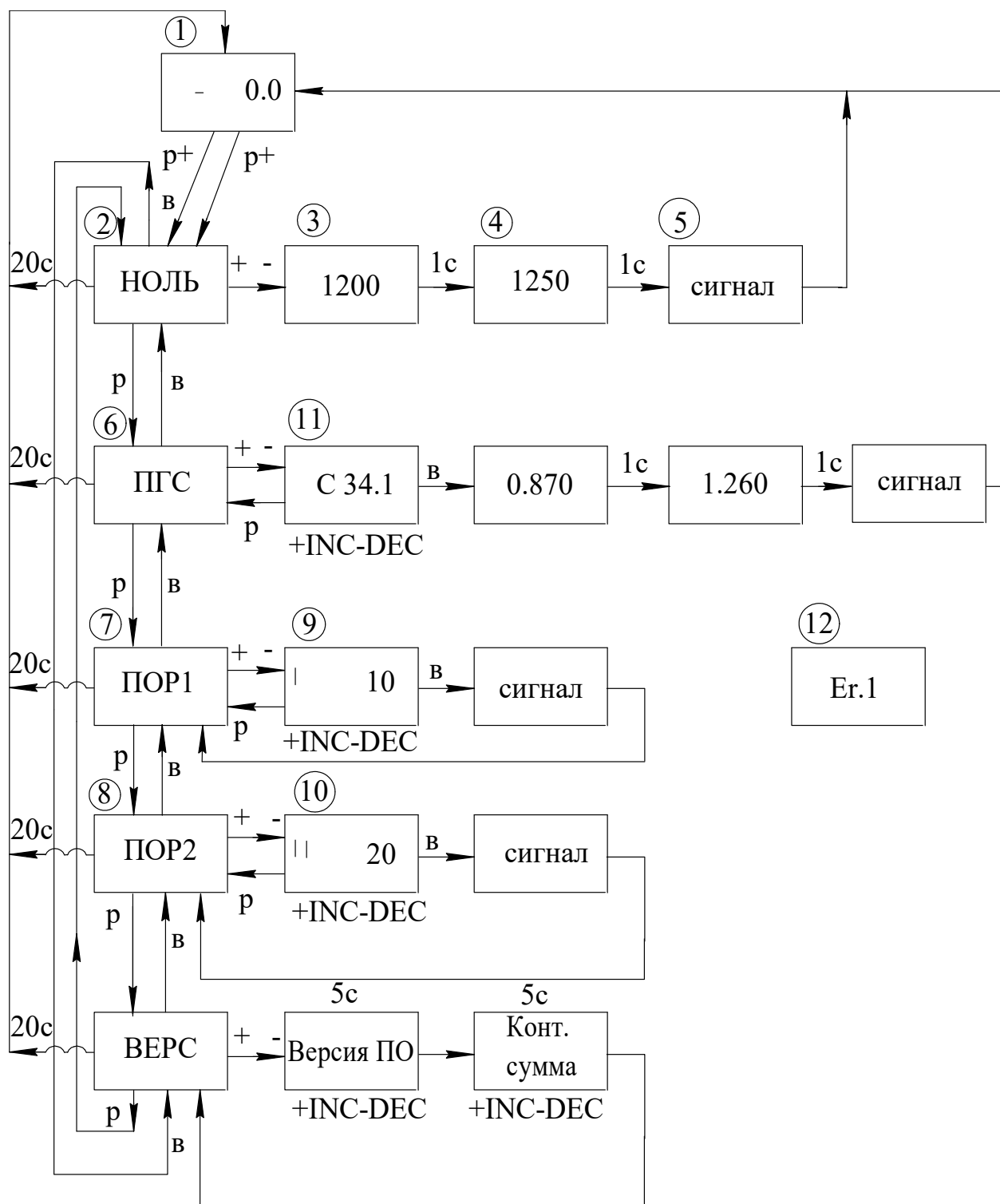
Рисунок Д.2 – БД. Алгоритм работы
